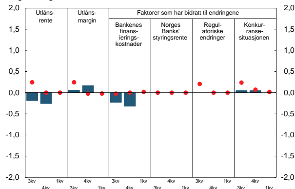
Figur 17 Utlånsrente og utlånsmargin. 1 Lån til ikke-finansielle foretak. Endring fra foregående kvartal. 2 3. kv. 2017 - 1. kv. 2018
