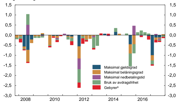
Figur 8 Lånebetingelser overfor husholdninger. 1 Endring fra foregående kvartal. 2 4. kv. 2007 - 4. kv. 2017
