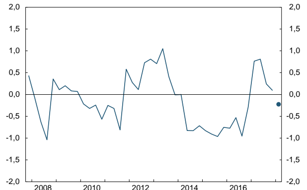
Figur 10 Utlånsmargin på samlede lån med pant i bolig til husholdninger. 1 Endring fra foregående kvartal. 2 4. kv. 2007 - 1. kv. 2018
