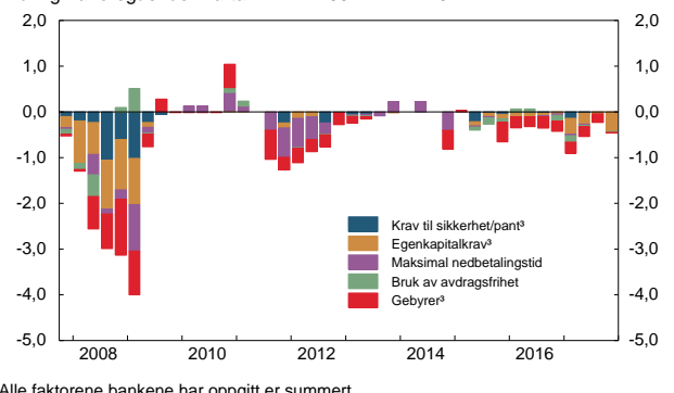
Figur 16 Lånebetingelser overfor ikke-finansielle foretak. 1 Endring fra foregående kvartal. 2 4. kv. 2007 - 4. kv. 2017
