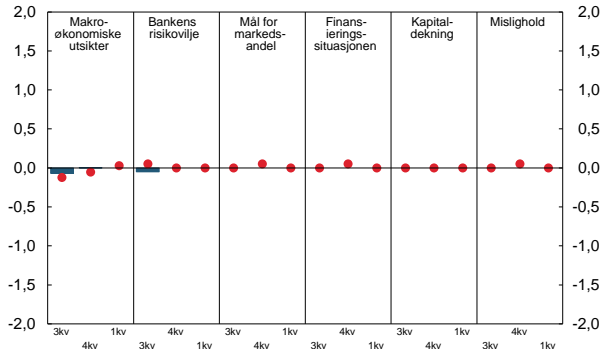
Figur 5 Faktorer som påvirker kredittpølsen overfor husholdninger. 1 Endring fra foregående kvartal. 2 3. kv. 2017 - 1. kv. 2018
