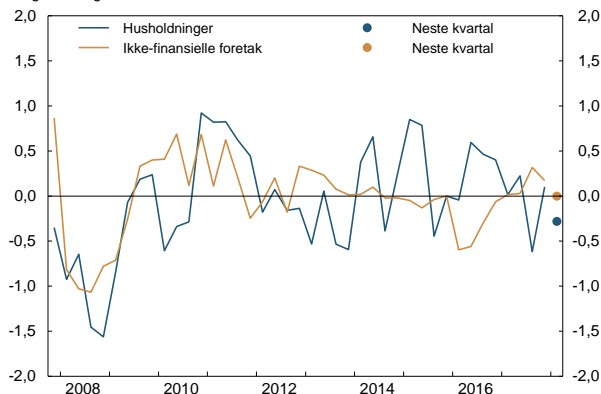
Figur 1 Etterspørsel etter lån fra husholdninger 1 og ikke-finansielle foretak 2 . Endring fra foregående kvartal. 3 4. kv. 2007 - 1. kv. 2018
