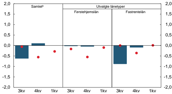
Figur 3 Husholdningenes etterspørsel etter lån med pant i bolig 1 . Endring fra foregående kvartal. 2 3. kv. 2017 - 1. kv. 2018
