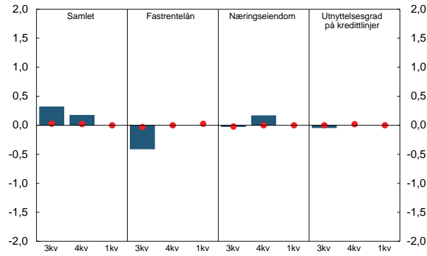
Figur 11 Etterspørsel etter lån fra ikke-finansielle foretak. 1 Endring fra foregående kvartal. 2 3. kv. 2017 - 1. kv. 2018
