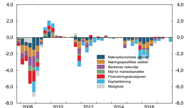
Figur 14 Faktorer som påvirker kredittpraksisen overfor ikke-finansielle foretak. 1 Endring fra foregående kvartal. 2 4. kv. 2007 - 4. kv. 2017
