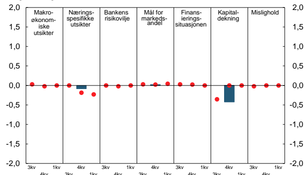
Figur 13 Faktorer som påvirker kredittpraksisen overfor ikke-finansielle foretak. 1 Endring fra foregående kvartal. 2 3. kv. 2017 - 1. kv. 2018
