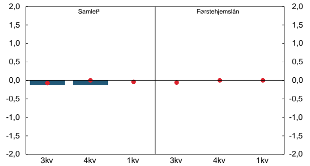
Figur 4 Kredittpølse overfor husholdninger. 1 Endring fra foregående kvartal. 2 3. kv. 2017 - 1. kv. 2018
