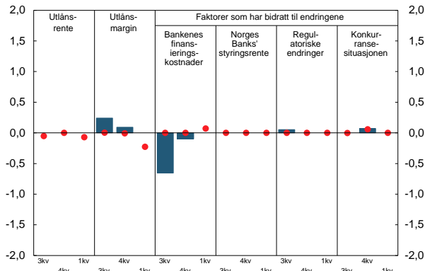
Figur 9 Utlånsrente og utlånsmargin. 1 Lån til husholdninger. Endring fra foregående kvartal. 2 3. kv. 2017 - 1. kv. 2018
