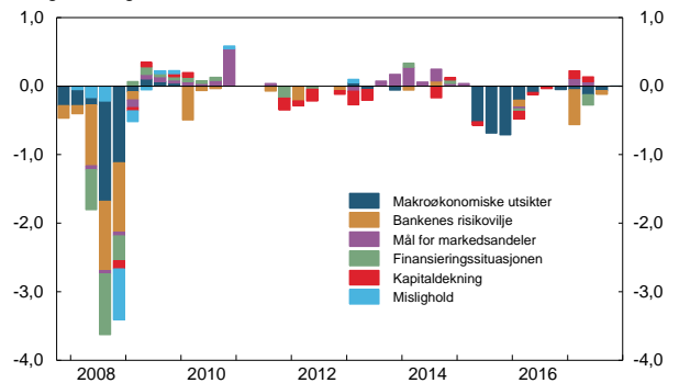
Figur 6 Faktorer som påvirker kredittpølsen overfor husholdninger. 1 Endring fra foregående kvartal. 2 4. kv. 2007 - 4. kv. 2017
