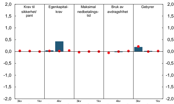
Figur 15 Lånebetingelser overfor ikke-finansielle foretak. 1 Endring fra foregående kvartal. 2 3. kv. 2017 - 1. kv. 2018
