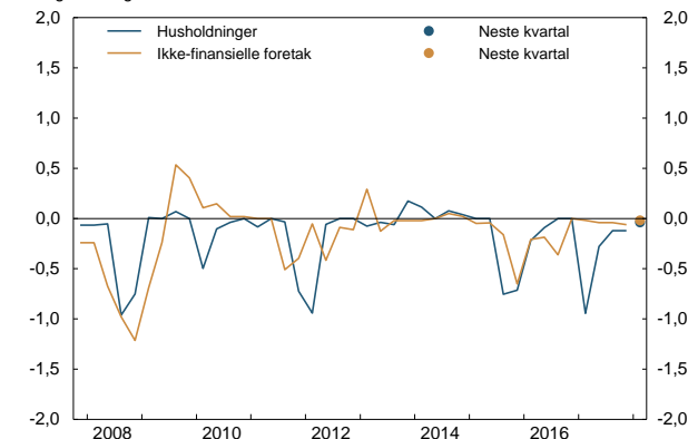
Figur 2 Kredittpraksis overfor husholdninger 1 og ikke-finansielle foretak 2 . Endring fra foregående kvartal. 3 4. kv. 2007 - 1. kv. 2018
