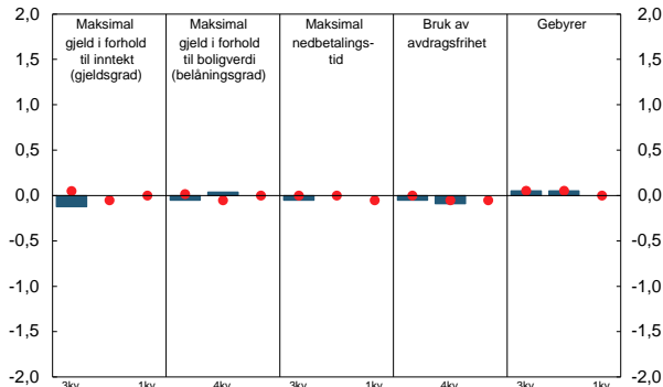
Figur 7 Lånebetingelser overfor husholdninger. 1 Endring fra foregående kvartal. 2 3. kv. 2017 - 1. kv. 2018
