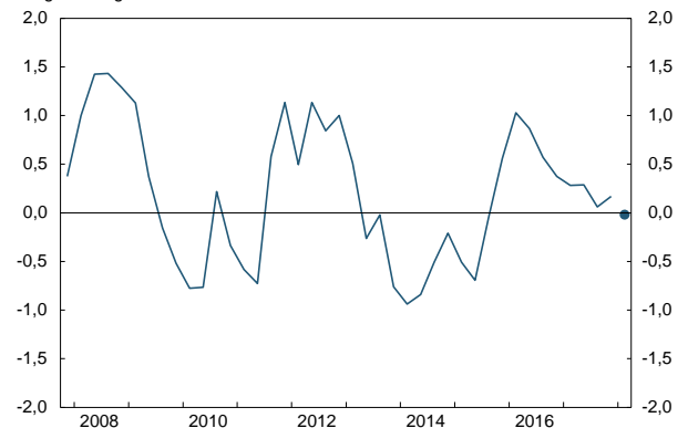
Figur 18 Utlånsmargin på samlede lån til ikke-finansielle foretak. 1 Endring fra foregående kvartal. 2 4. kv. 2007 - 1. kv. 2018
