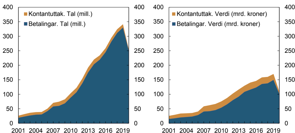
Figur 10 Bruk av norske betalingskort mot utlandet. 2001–2020
