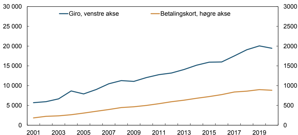
Figur 2 Bruk av betalingsinstrument. Milliardar kroner. 2001–2020
