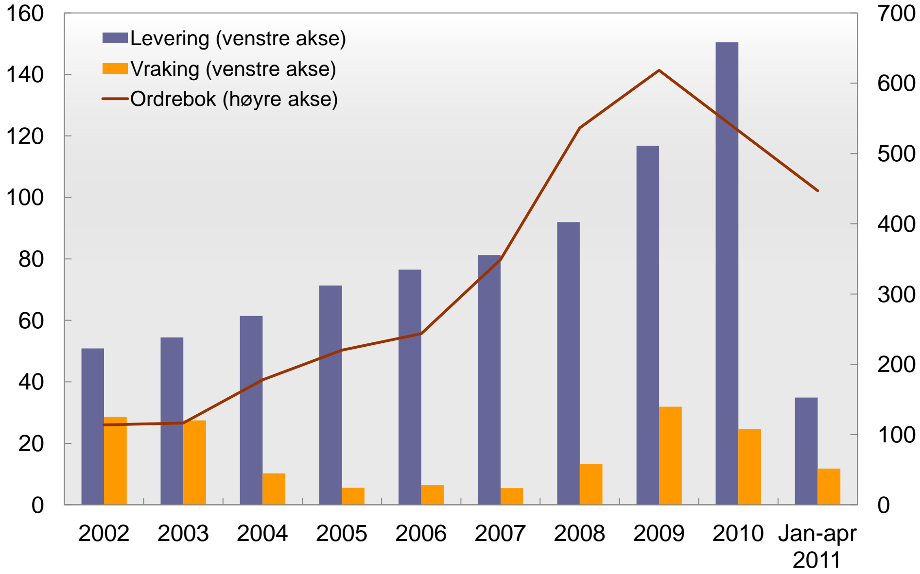
Figur 1.34 Ordrer, levering og vraking av skip på verdensbasis. Millioner dødvekttonn. Månedstall. 2002 – 2011
